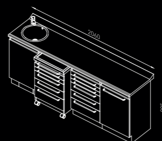
Composizione 4 elementi con lavello inox e servomobile. Run of 4 cabinets with stainless steel sink and mobile cabinet.
